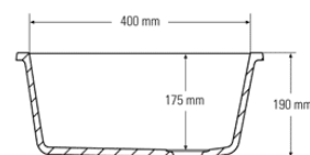
Querschnitt Seitenansicht
