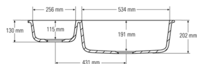
Querschnitt Seitenansicht
