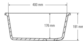
Querschnitt Seitenansicht
