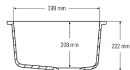
Querschnitt Seitenansicht
