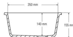
Querschnitt Seitenansicht
