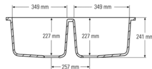
Querschnitt Seitenansicht
