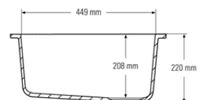
Querschnitt Seitenansicht
