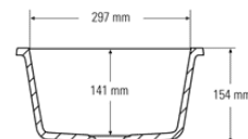
Querschnitt Seitenansicht
