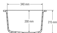
Querschnitt Seitenansicht
