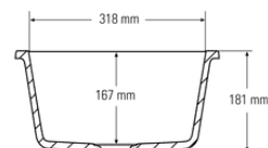
Querschnitt Seitenansicht
